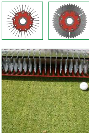
TERRA FLOAT mit Nachsaateinheit | TERRA FLOAT with reseed unit | TERRA FLOAT avec unité de regarnissage
